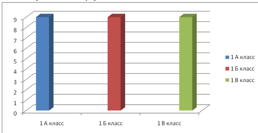
Гистограмма данных
