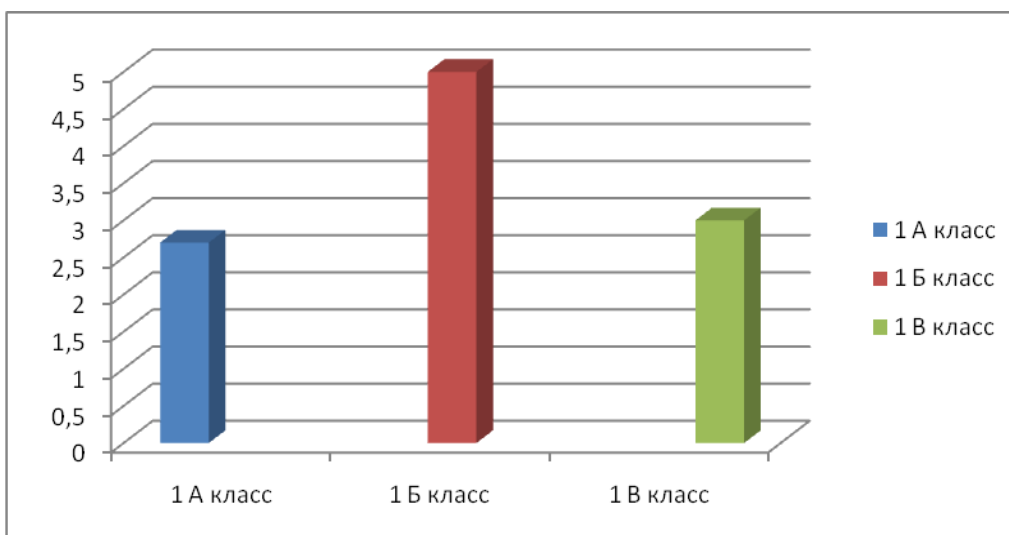
Гистограмма данных
