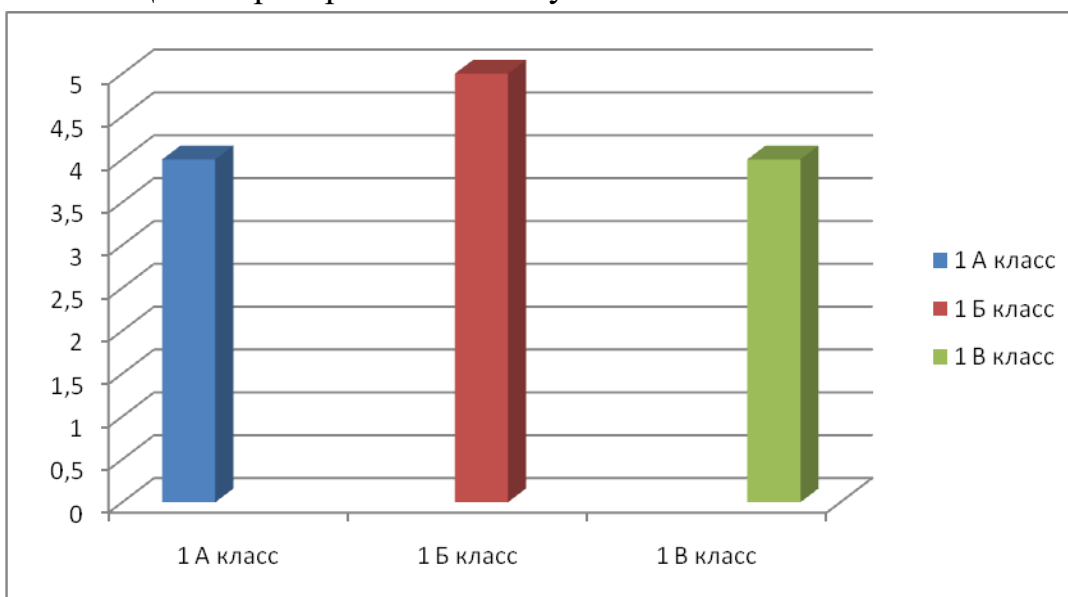
Гистограмма данных
