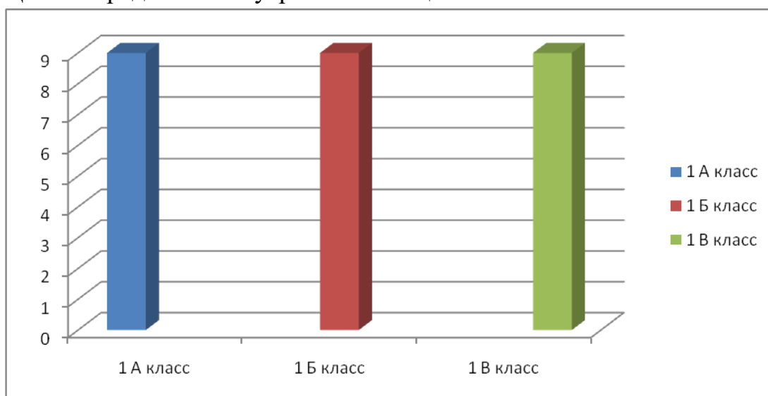
Гистограмма данных
