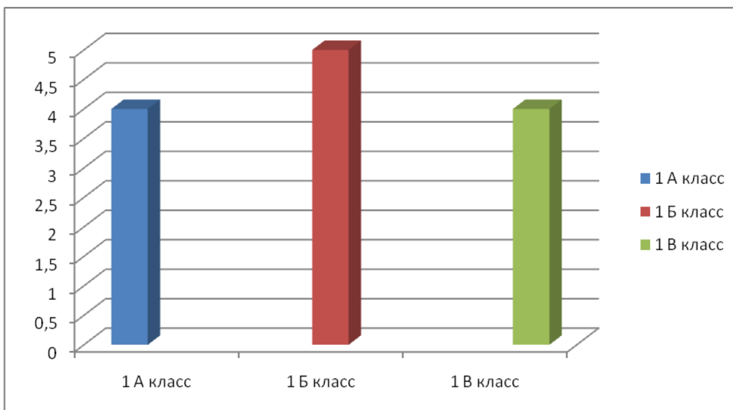
Гистограмма данных
