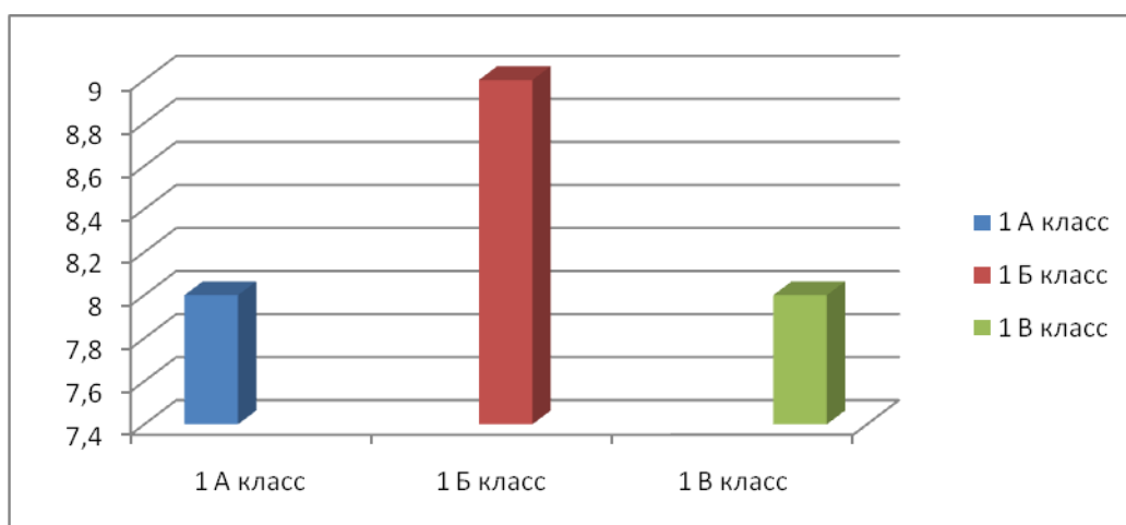
Гистограмма данных
