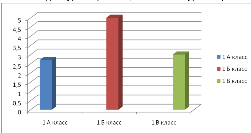
Гистограмма данных
