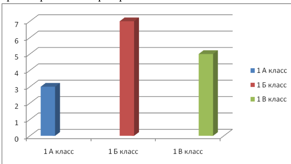
Гистограмма данных
